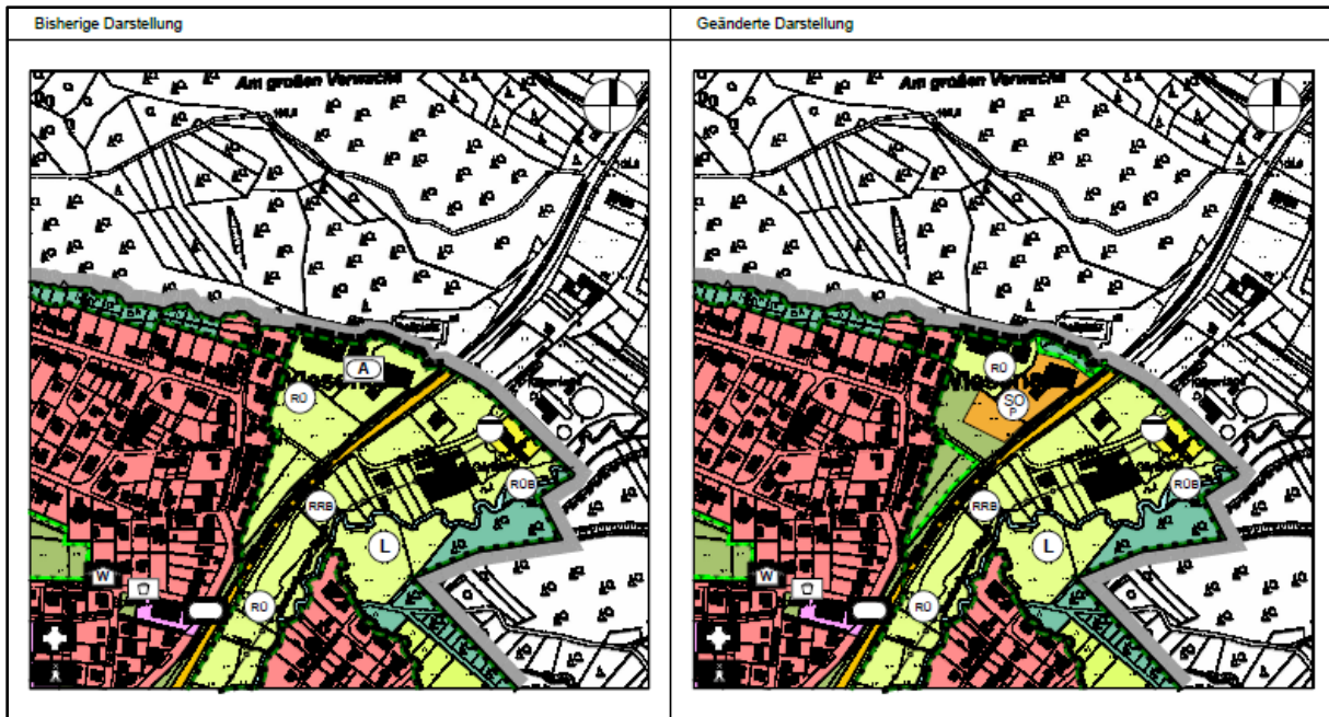
Abbildung 2: Auszug aus der Plandarstellung zur 2. Änderung des Flächennutzungsplans (NAUMANN, Stand 08.08.2023)
